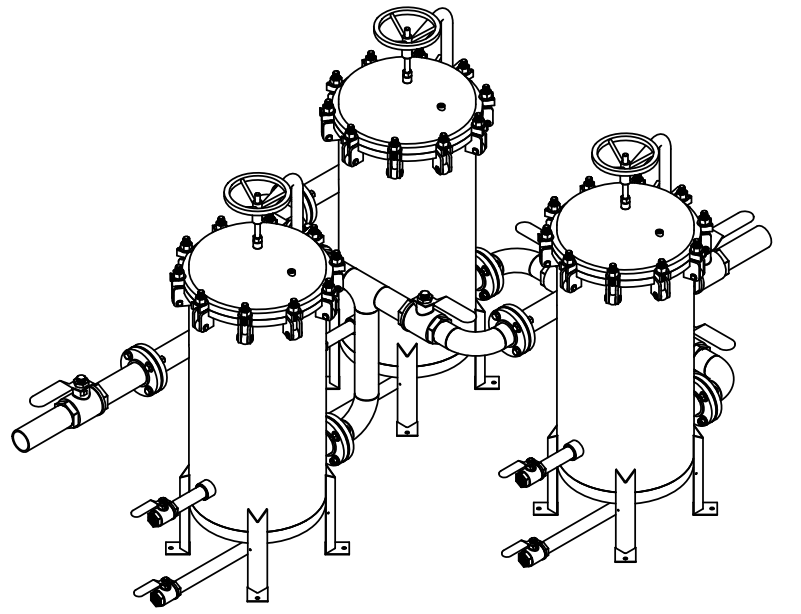
ИЗОМЕТРИЧЕСКИЙ ВИД
